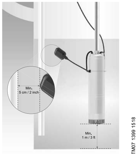
Рис. 6 Минимальное пространство для насоса SB HF. В данном примере монтаж показан в скважине
